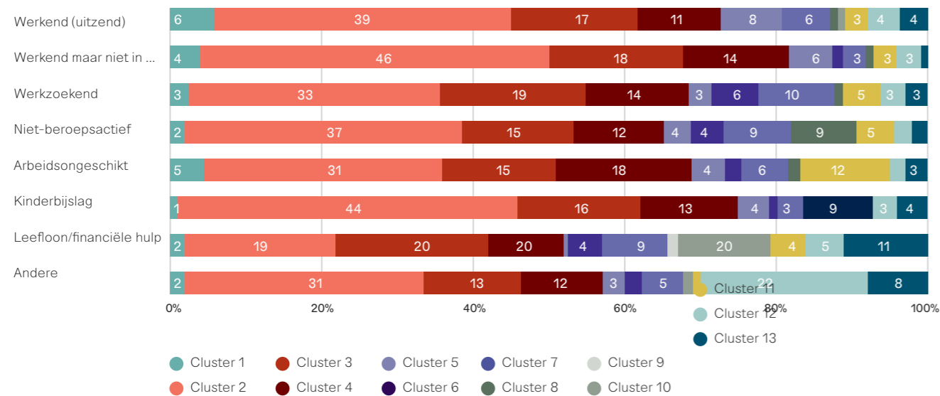
Figuur 6 - Sequentie-analyse 1:
